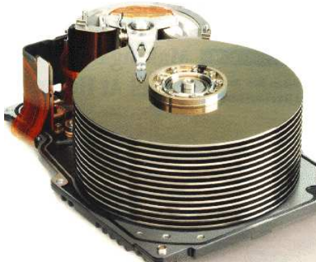
Figura: Disco magnético
