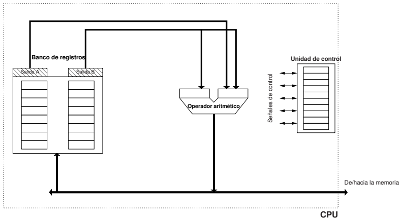
Figura: Estructura interna de la CPU
