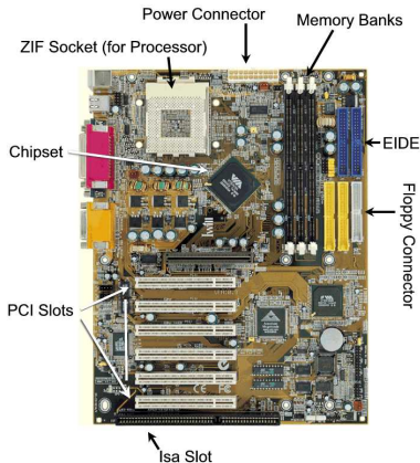
Figura: Placa madre
