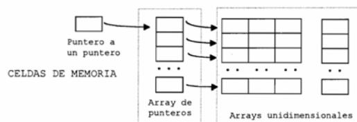
ARRAY BIDIMENSIONAL CREADO MEDIANTE ASIGNACIÓN DINÁMICA DE MEMORIA
